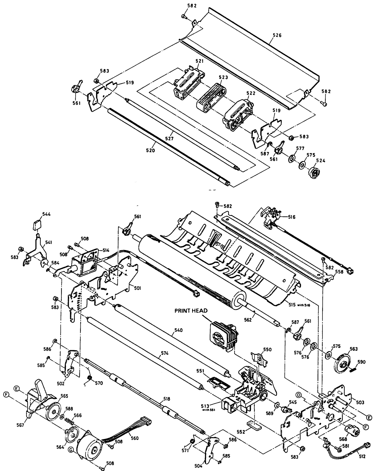
FX850 FIG.2
