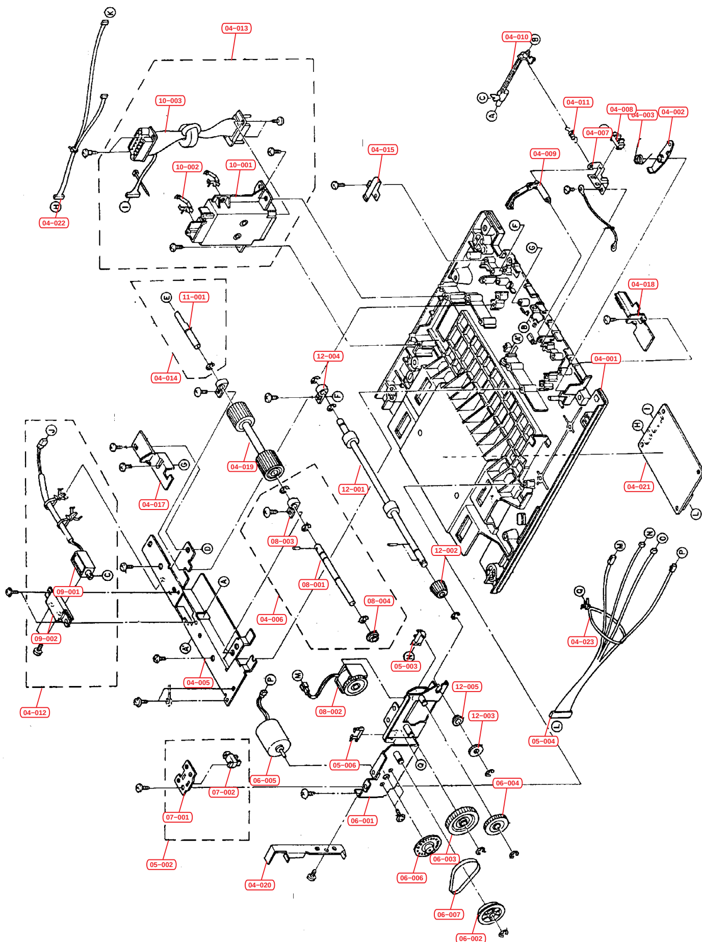
Fig.3 – Partie supérieure
