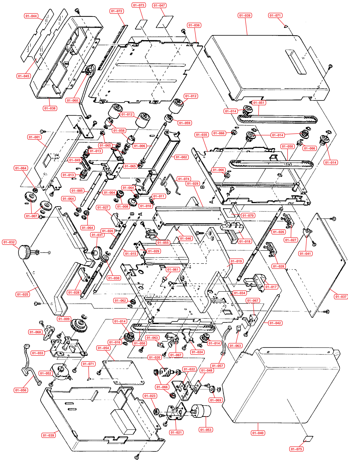
Fig.1 – Mécanisme entrainement papier PF-7
